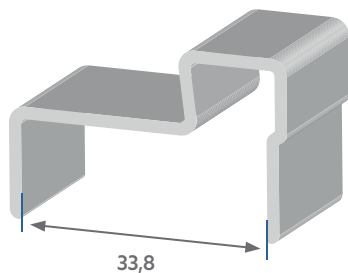
R 9009 | Perfil para montagem de divisória
