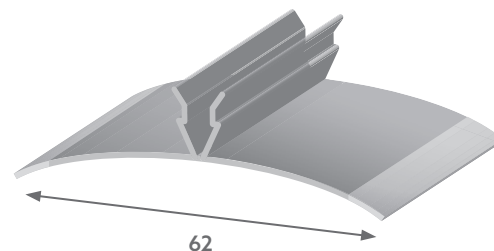
R 3072 | Acabamento de sobrepor 62 mm c/ co-extrusão
