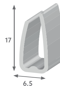
R 3032 | Perfil para acabamento de chapas de PC 17x6,5
