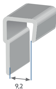
R 9010 | Perfil para montagem de divisória
