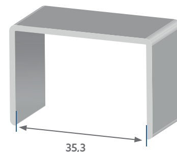
R 9023 | Perfil para montagem de divisória
