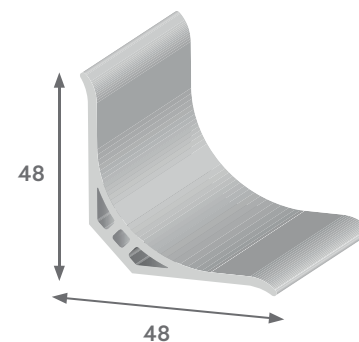
F 4084 | Rodapé | Sala limpa | Canto interno
