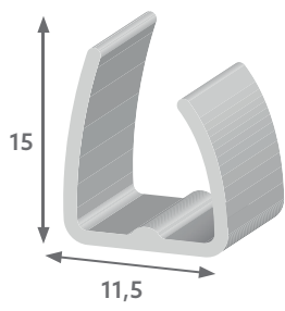
R 3033 | Perfil para acabamento de chapas de PC 15x11,5
