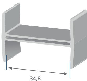
R 9026 | Perfil para montagem de divisória
