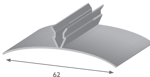
R 2384 | Acabamento de sobrepor 62 mm
